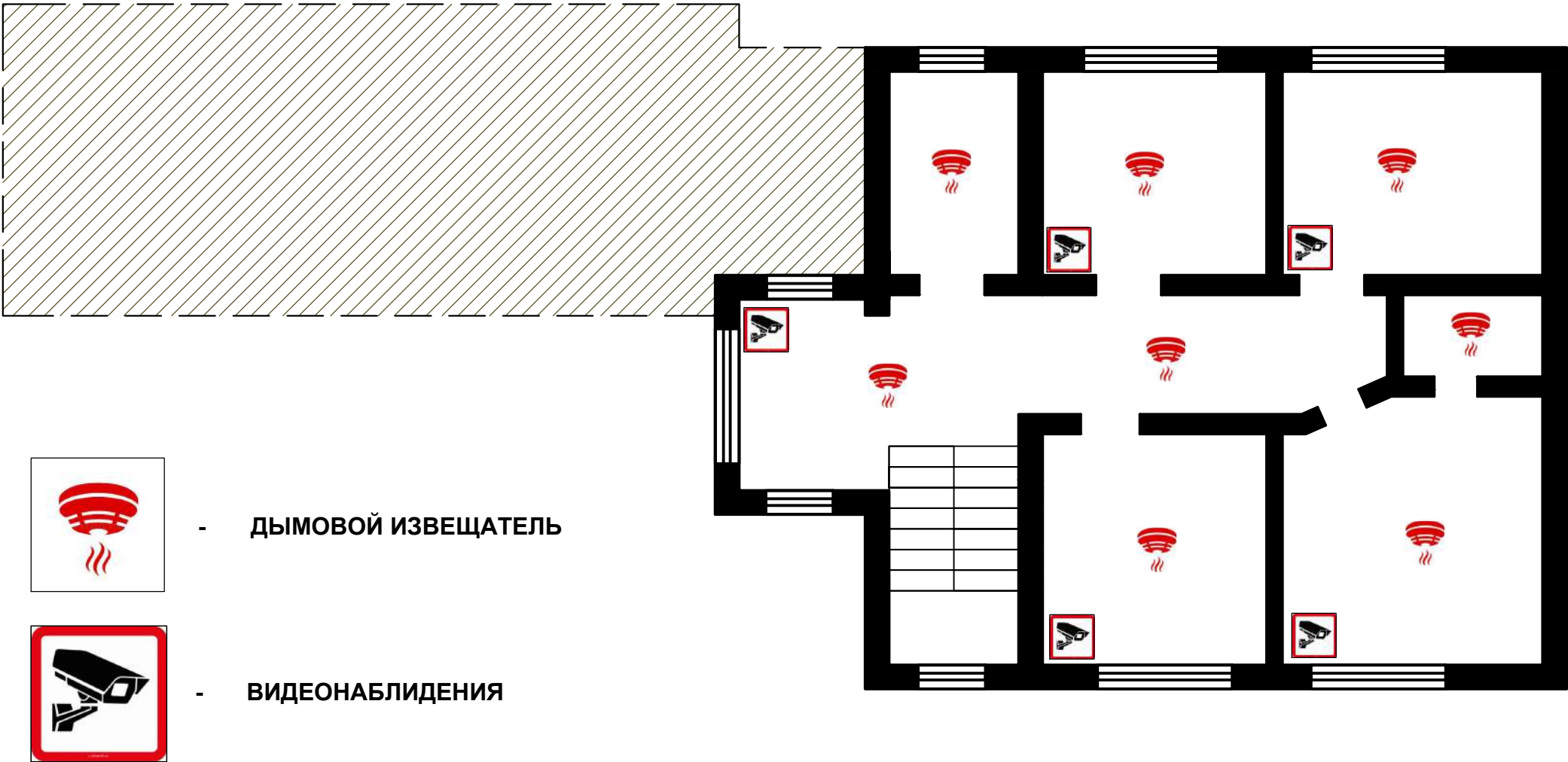
ПЛАН ВИДЕОНАБЛИДЕНИЯ И ДЫМОВЫХ ИЗВЕЩАТЕЛЕЙ 2-ГО ЭТАЖА
