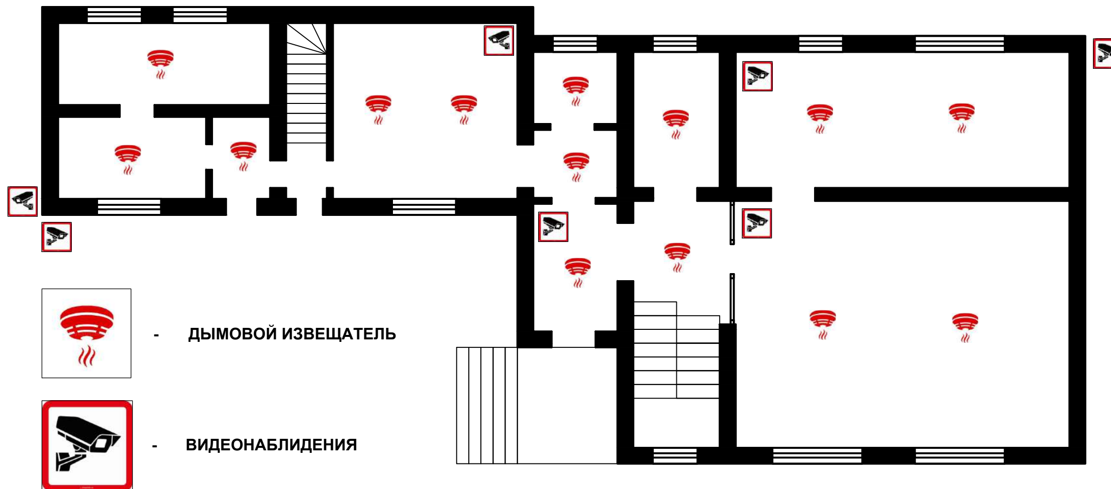
ПЛАН ВИДЕОНАБЛИДЕНИЯ И ДЫМОВЫХ ИЗВЕЩАТЕЛЕЙ 2-ГО ЭТАЖА
